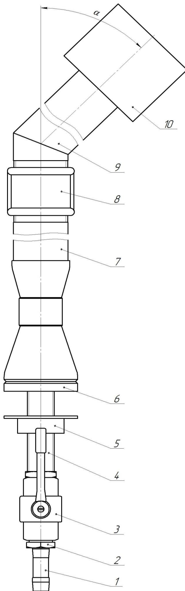
Рисунок 1 – Горелка МП-ГВИ-2
